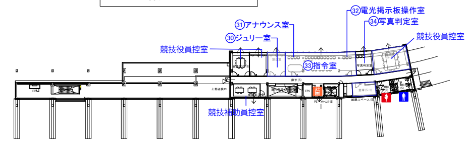
4階 平面図
